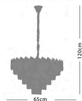
Kod 3090-65-F 15 x E14
