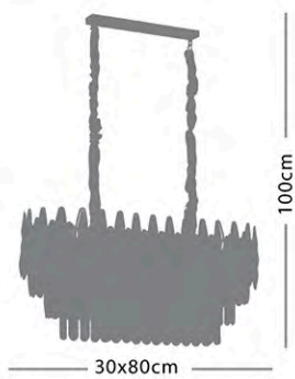
Kod 3042-YM-K 10 x E14
