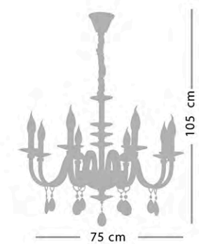
Kod 8698-8 8 x E14
