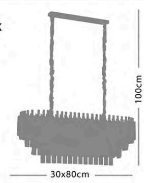
Kod 3002-YM-K 10 x E14
