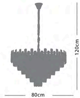
Kod 3035-80-F 20 x E14
